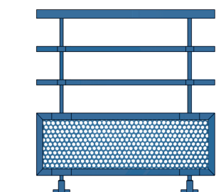
Paquebot à remplissage tôle perforée avec 2 tubes Ø30
