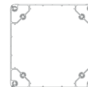
poteau à sceller de section 200x200mm
