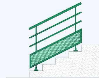
Rampant remplissage tôle perforée avec 2 tubes Ø30
