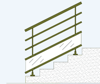
Rampant remplissage verre avec 2 tubes Ø30
