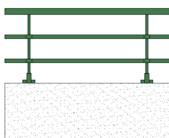
Paquebot avec 2 tubes Ø30 sur muret (hauteur mini du muret 450mm)
