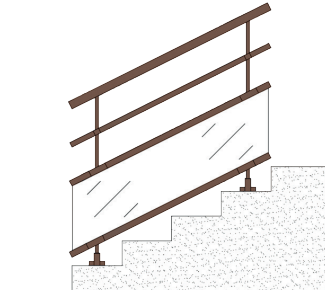
Rampant remplissage verre avec 1 tube Ø30
