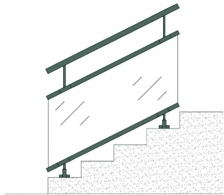
Rampant remplissage verre
