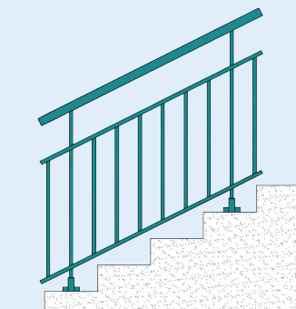
Rampant barreaudé avec lisse intermediaire
