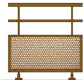
Paquebot à remplissage tôle perforée avec 1 tube Ø30
