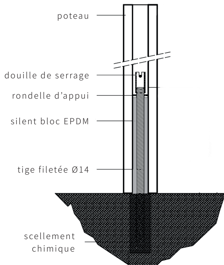
FIXATION DIODON (modèle breveté)
