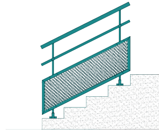
Rampant remplissage tôle perforée avec 1 tube Ø30
