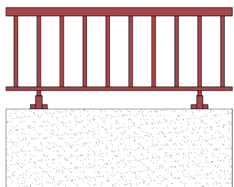
A barreauté sur muret (hauteur mini du muret 450mm)
