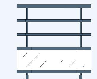
Paquebot à remplissage verre avec 2 tubes Ø30
